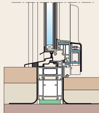
Detail met low-step en Nova-line deur
