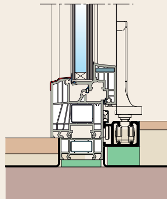
Detail kunststof onderdorpel
