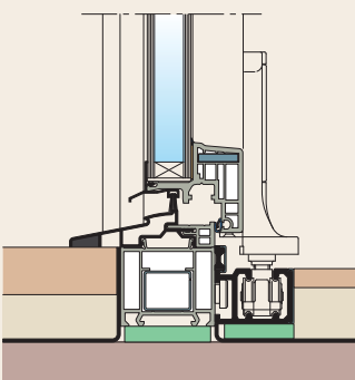
Detail aluminium onderdorpel
