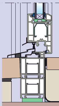
Aluminium onderdorpel
