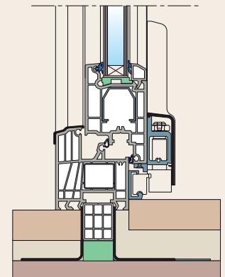
Detail met kunststof onderdorpel (standaard)
